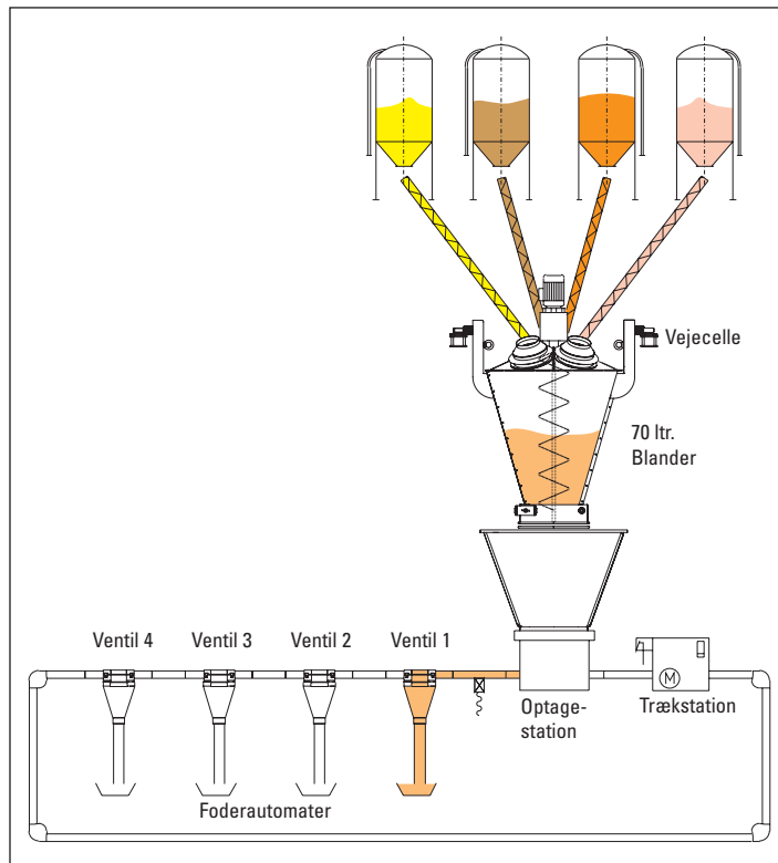
Processkema over DRY EXACT anlægget
